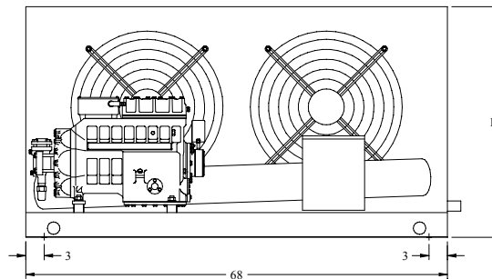
FRONT VIEW - 2 FAN MODEL DE
