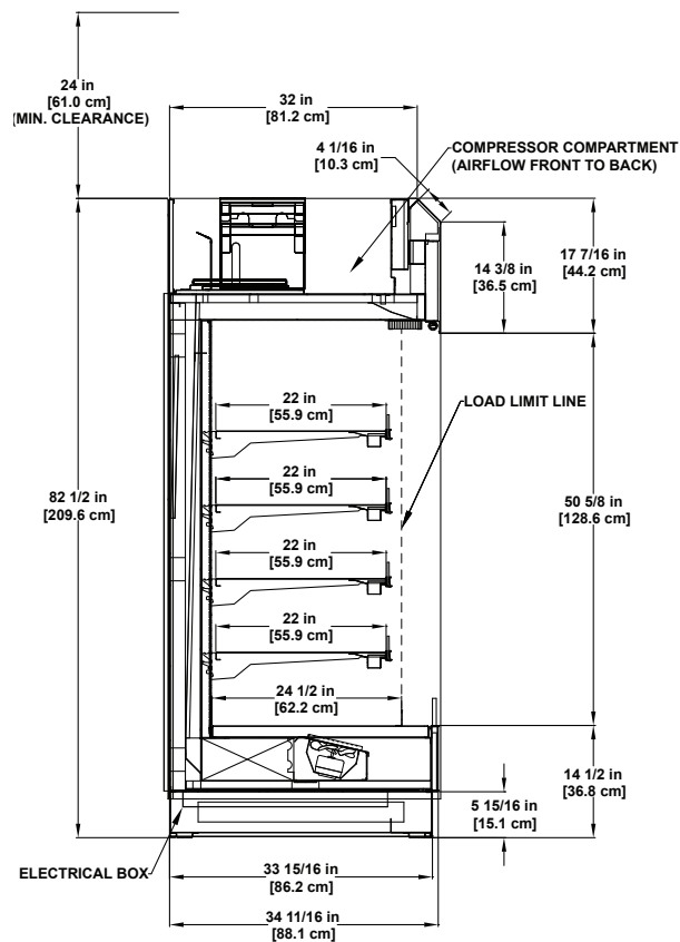
QTM-35 Refrigerated 36", 47", 68", 72", 95", 120" & 143" Multi-deck Display
