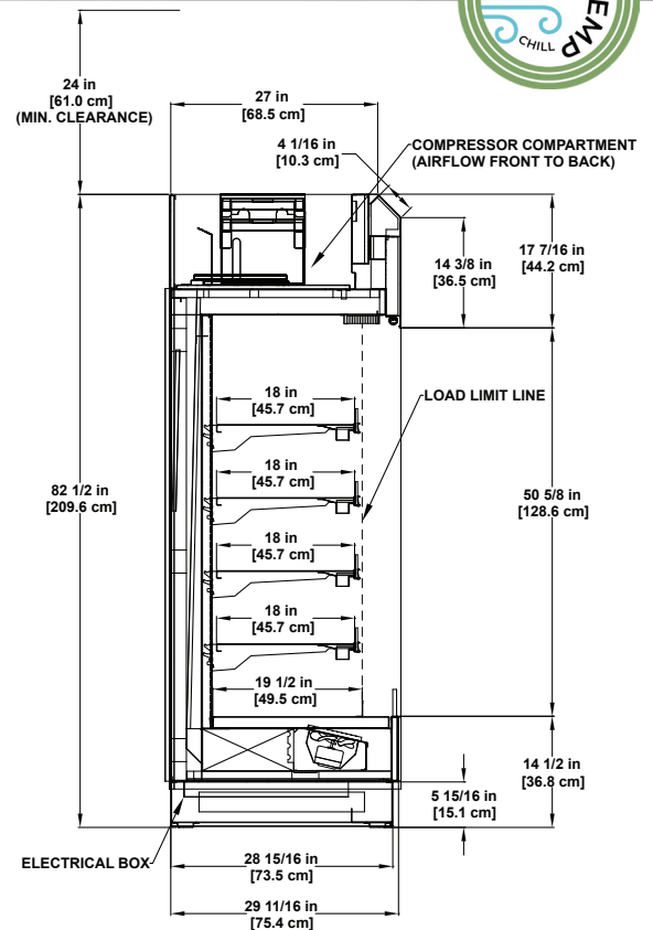
QTM-30 Refrigerated 36", 47", 68", 72", 95", 120" & 143" Multi-deck Display
