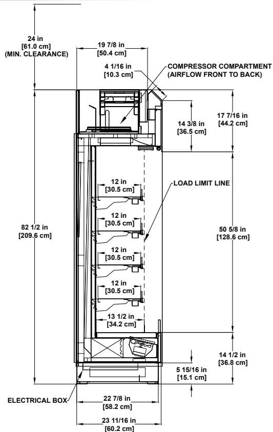
QTM-24 Refrigerated 36", 47", 68", 72", 95", 120" & 143" Multi-deck Display
